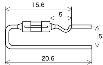
フォーミング No. F006
