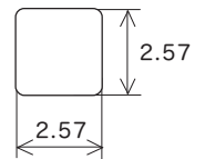
リフローはんだランドパターン (参考寸法)
