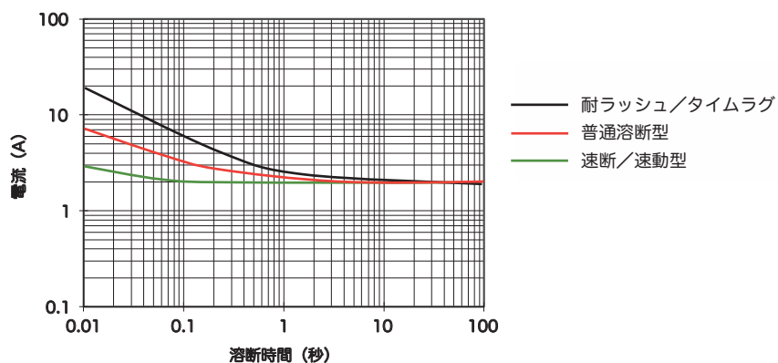
【図 7】 同じ定格電流での溶断特性による溶断時間-電流特性の違い (イメージ図)
