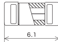
リフローはんだランドパターン (参考寸法)
