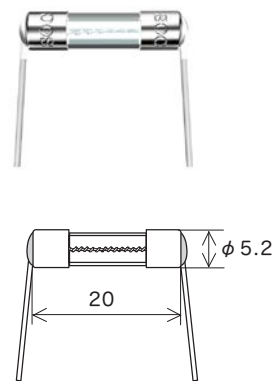
リード線径 \phi 0.8 (3.5A 超 ~ 10A) 倍率 1/1 \phi 1.0 (10A 超 ~ 15A) (mm)
