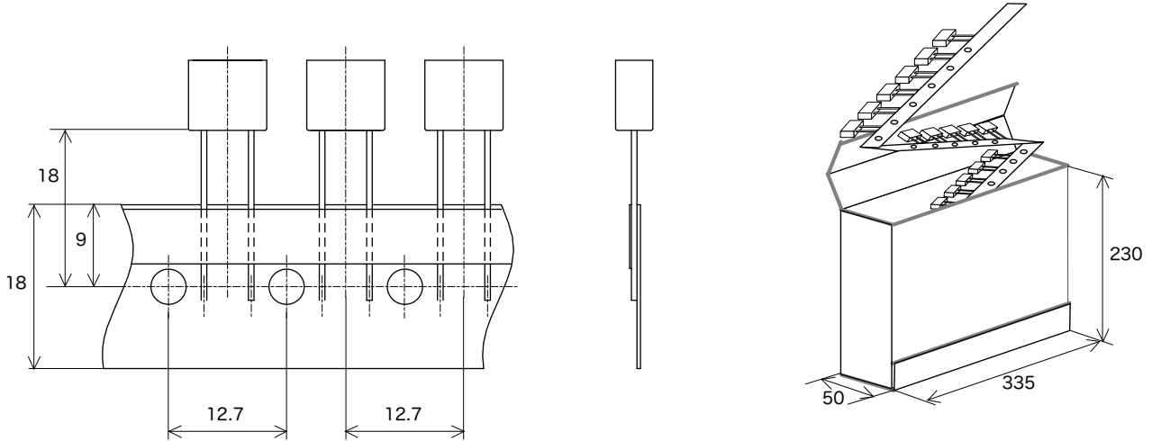
SMC N4 テーピング形状 / 包装形態 (単位: mm)
