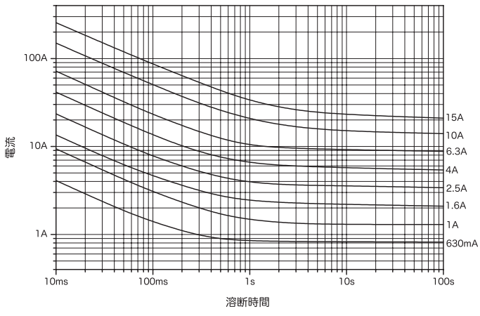
代表的な溶断時間-電流特性 (参考)
