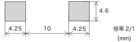
リフローはんだランドパターン (参考寸法)
