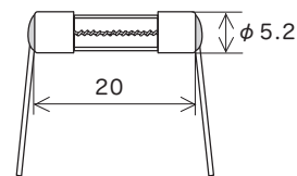
リード線径 φ 0.5 (100mA ~ 5A 未満) φ 0.8 (5A ~ 10A) 倍率 1/1 (mm)
