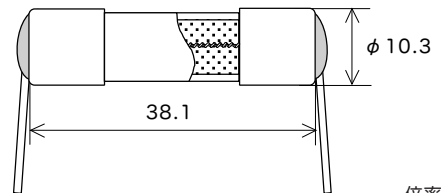
リード線径 φ 1.2 倍率 1/1 (mm)
