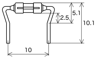
フォーミング No. F007
