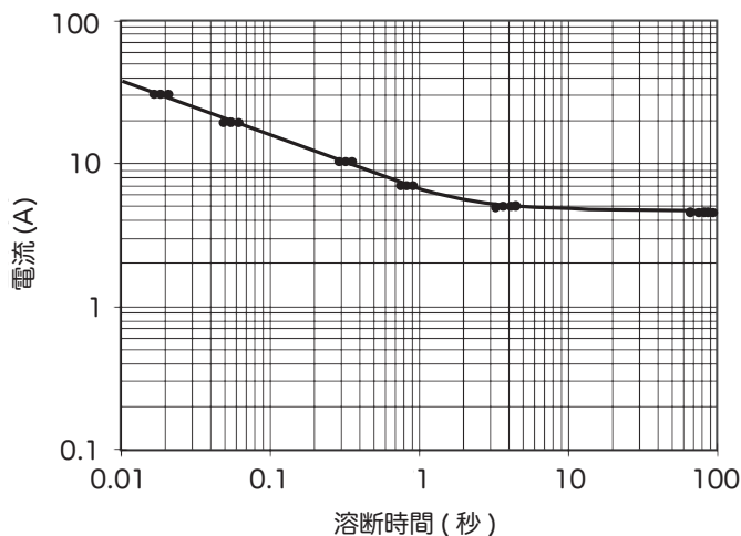
【図3】 溶断時間-電流特性の作成例
