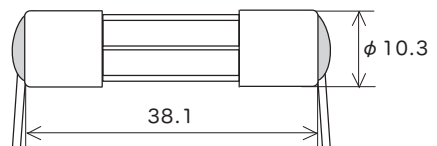
リード線径 φ 0.8 (500mA ~ 8A) φ 1.0 (8A 超 ~ 15A) φ 1.2 (15A 超 ~ 30A)
