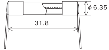
リード線径 φ 0.8 (100mA ~ 8A) φ 1.2 (8A 超 ~ 25A) 倍率 1/1 (mm)
